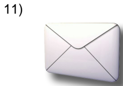
e-mail
