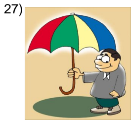
default option
